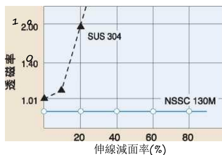
〔透磁率〕伸線加工後透磁率
